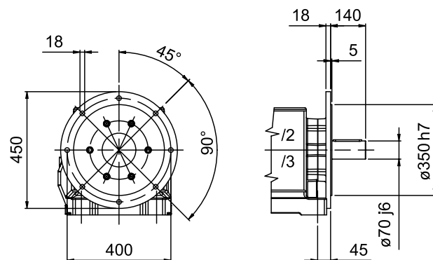
EINGEBAUTER FLANSCH
