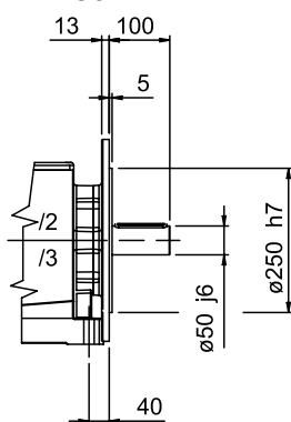
EINGEBAUTER FLANSCH
