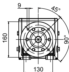
MODULAR FLANGE
