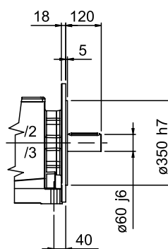
EINGEBAUTER FLANSCH
