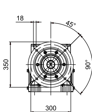
FLANGIA RIPORTATA
