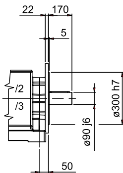
MODULAR FLANGE
