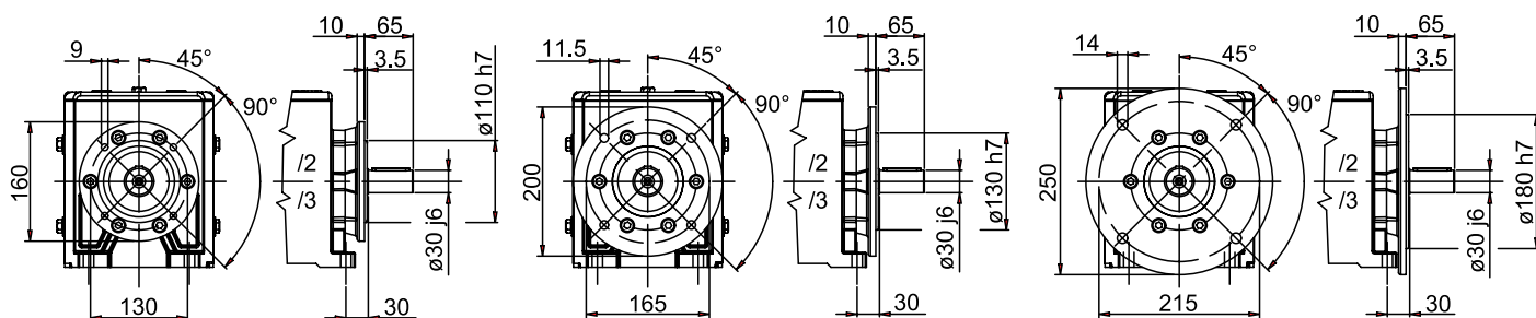
FLANGIA RIPORTATA
