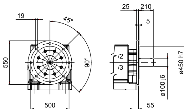
MODULAR FLANGE
