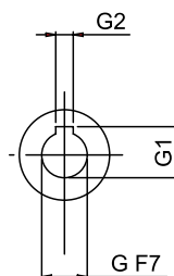
ALBERO ENTRATA INPUT SHAFT ANTRIEBSWELLE
