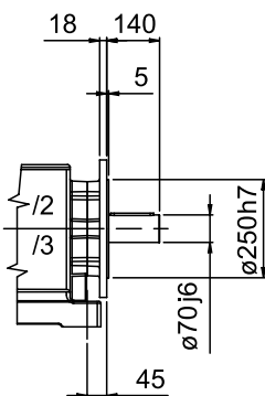
MODULAR FLANGE
