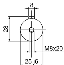
ALBERO USCITA OUTPUT SHAFT ABTRIEBSWELLE
