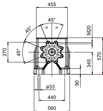
FLANGIA RIPORTATA
