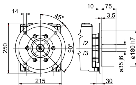
EINGEBAUTER FLANSCH
