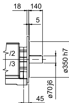
EINGEBAUTER FLANSCH
