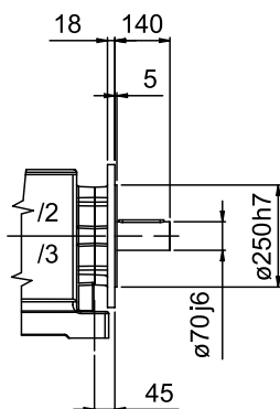
MODULAR FLANGE
