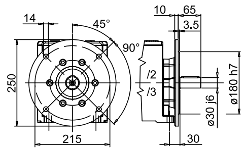
EINGEBAUTER FLANSCH
