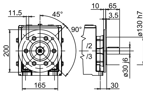
MODULAR FLANGE
