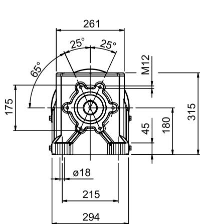
FLANGIA RIPORTATA
