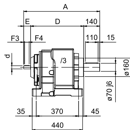
NHL 70 - GETRIEBE
