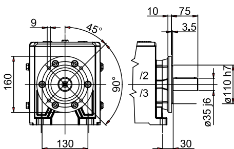
FLANGIA RIPORTATA
