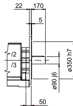
EINGEBAUTER FLANSCH
