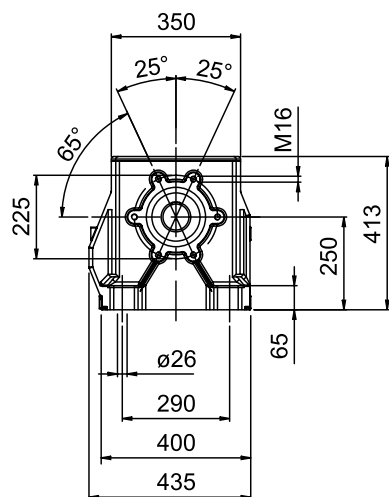
FLANGIA RIPORTATA
