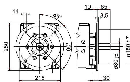
EINGEBAUTER FLANSCH
