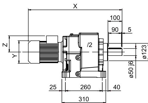
MODULAR FLANGE
