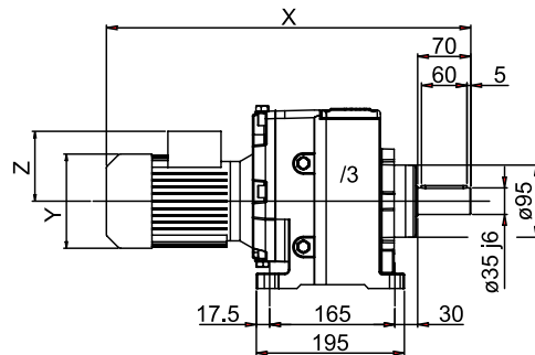
EINGEBAUTER FLANSCH
