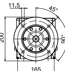
EINGEBAUTER FLANSCH
