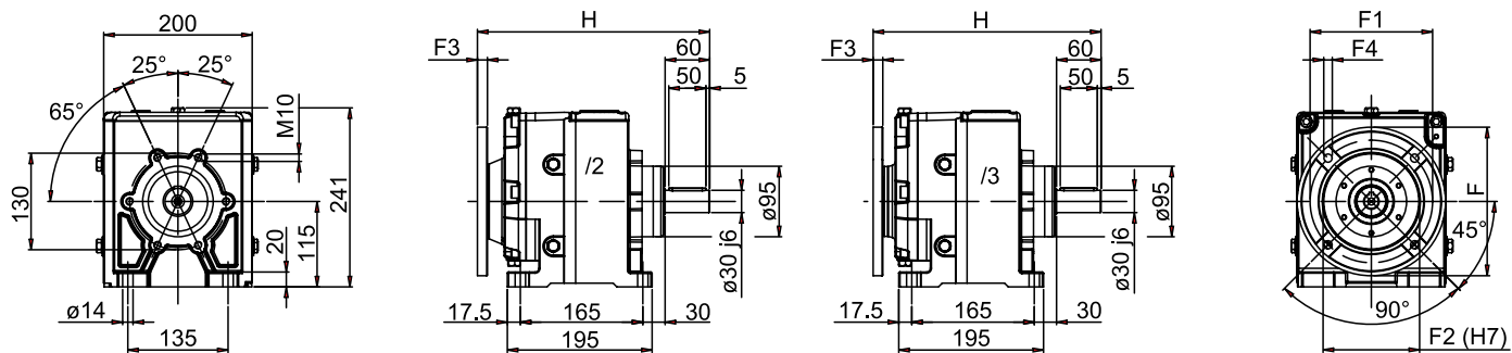
FLANGIA RIPORTATA
