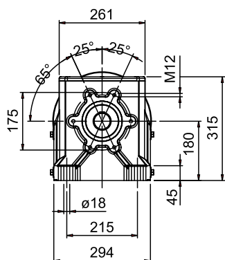
FLANGIA RIPORTATA
