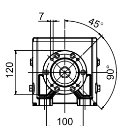
FLANGIA RIPORTATA
