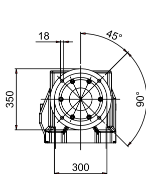
FLANGIA RIPORTATA
