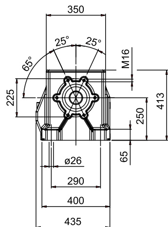
FLANGIA RIPORTATA
