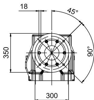
FLANGIA RIPORTATA
