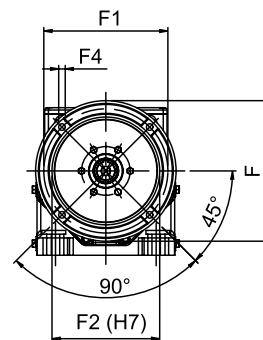
EINGEBAUTER FLANSCH
