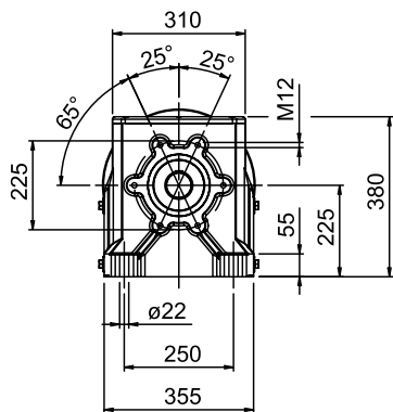
FLANGIA RIPORTATA
