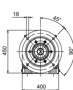
EINGEBAUTER FLANSCH
