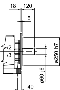
MODULAR FLANGE
