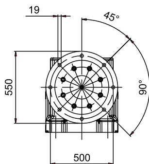
MODULAR FLANGE
