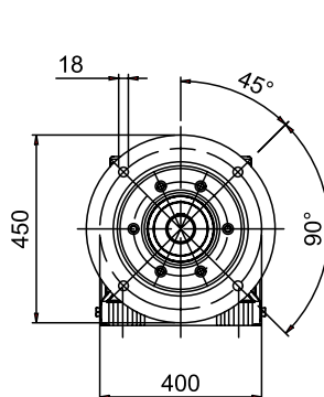
EINGEBAUTER FLANSCH
