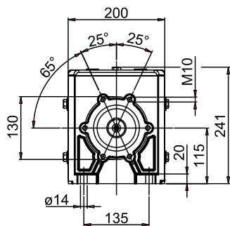
FLANGIA RIPORTATA
