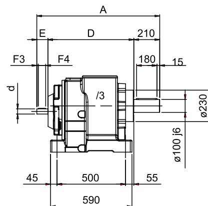
EINGEBAUTER FLANSCH
