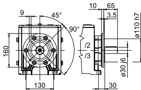
FLANGIA RIPORTATA
