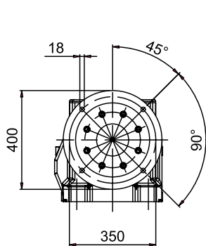
FLANGIA RIPORTATA
