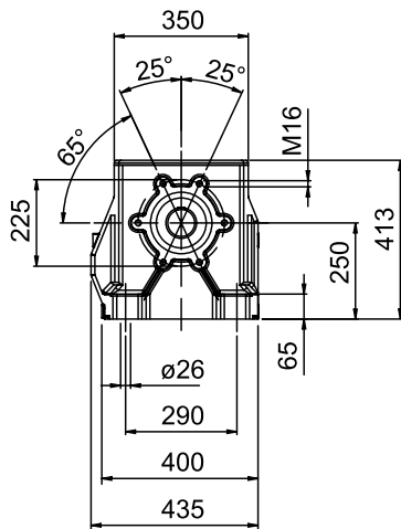
FLANGIA RIPORTATA
