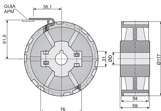
Piñón Z19 Cadena Recta Inox. Con Chavetero Tipo 815-812... Sprockets Z19 Straight Stainless Chain Type 815-812 With Keyway
