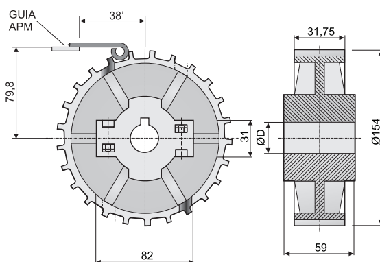
Piñón Z25 Cadena Curva Con Chavetero Tipo 881... Sprockets Z25 Curve Chain Type 881 With Keyway
