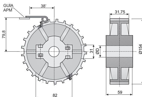
Piñón Z25 Cadena Curva Sin Chavetero Tipo 881... Sprockets Z25 Curve Chain Type 881
