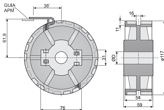
Piñón Z19 Cadena Recta Acetal Sin chavetero Tipo 820-831... Sprockets Z19 Straight Acetal Chain Type 820-831
