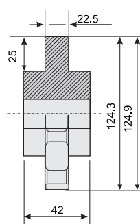
Piñón Z10 Cadena Curva Acetal Con Chavetero Tipo 882... Sprockets Z10 Curve Acetal Chain Type 882 With Keyway
